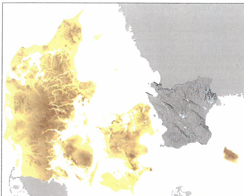
Fig. 7. Forsøg på kombineret terrænmodelkort for Danmark og Skåne. I den gul-brune danske del er fokus lagt på højdeforskelle, således at mørk farve viser højtliggende terræn; herved fremhæves bl.a. den jyske højderyg og de nordøstjyske ådale. I den metalgrå skånske del er fokus lagt på terrænets relief, hvor skyggelægningen illuderer en solindstråling fra sydvest; herved bliver den diagonale orientering (nordvest-sydøst) i det skånske terræn tydelig. Baseret på KMS' digitale terrænmodelkort (Dms 50) og Lantmäteriverkets digitala höjddatabas, sidstnævnte her indskannet og indsat fra Germundsson & Schlyter 1999, s. 17.
